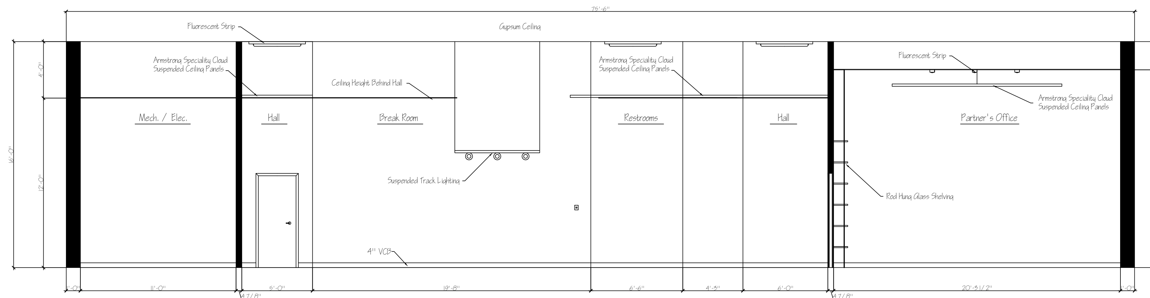
A LONGITUDINAL SECTION SCALE: 1/4" = 1'-0"
